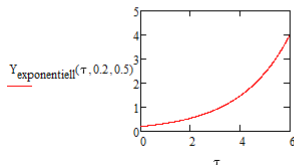
Abbildung 1: Exponentielles Wachstum (vgl. a. [SoA05,2])
