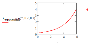
Abbildung 1: Exponentielles Wachstum
