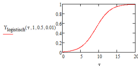
Abbildung 2: Logistische Kurve
